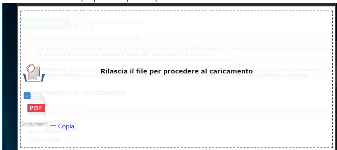
Figura 3 - File trascinato
