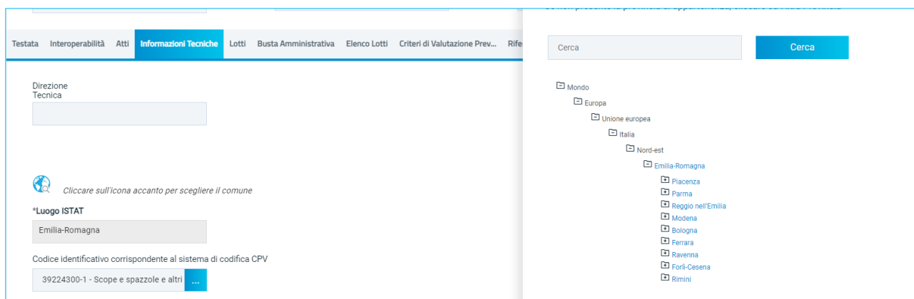
Figura 7 - Luogo istat
