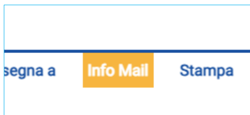
Figura 12 - Info Mail
