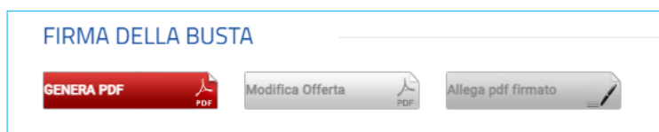
Figura 5 - Genera PDF
