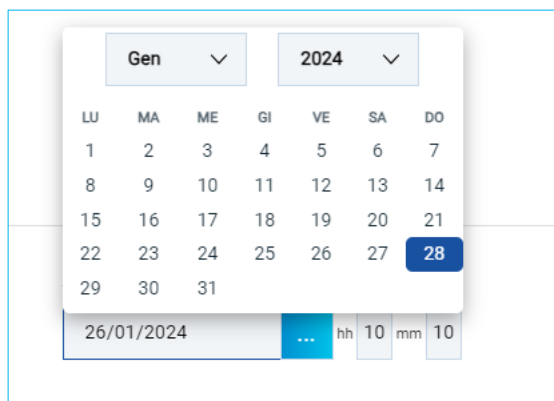
Figura 6 - Selezione date
